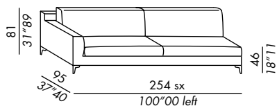
terminale / end unit 255
