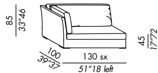
terminale / end unit 130
