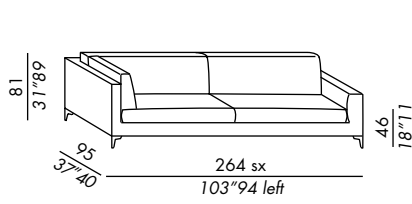
terminale angolo / corner end unit 265
